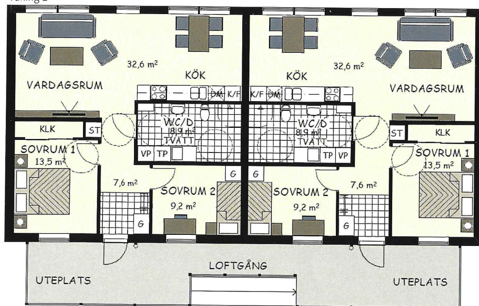
Våning 1
