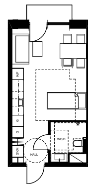
1 ROK 28,2m 2 MODULLÄNGD 7800mm MODULHÖJD 2850mm
