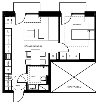
2 ROK 42,8 MODULLÄNGD 7310mm MODULHÖJD 2850mm
