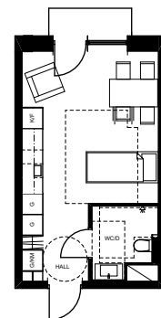
1 ROK 26,2m 2 MODULLÄNGD 7310mm MODULHÖJD 2850mm
