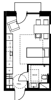
1 ROK 26,4m 2 (MED FÖNSTER I GAVELLÄGE) MODULLÄNGD 7310mm MODULHÖJD 2850mm
