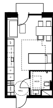
1 ROK 27,4m 2 MODULLÄNGD 7600mm MODULHÖJD 2850mm
