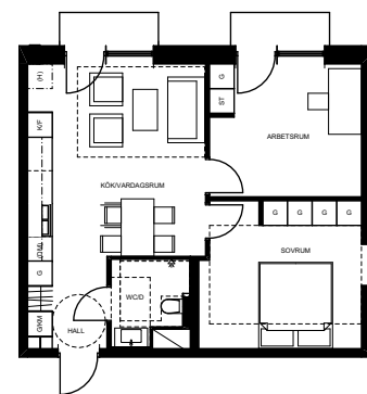
3 ROK 56,5m 2 MODULLÄNGD 7600mm MODULHÖJD 2850mm
