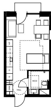
1 ROK 28,4m 2 (MED FÖNSTER I GAVELLÄGE) MODULLÄNGD 7800mm MODULHÖJD 2850mm
