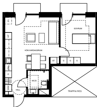
2 ROK 45,2m 2 MODULLÄNGD 7600mm MODULHÖJD 2850mm
