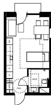
1 ROK 27,6m 2 (MED FÖNSTER I GAVELLÄGE) MODULLÄNGD 7600mm MODULHÖJD 2850mm
