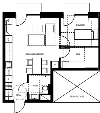
2 ROK 46,8m 2 MODULLÄNGD 7800mm MODULHÖJD 2850mm
