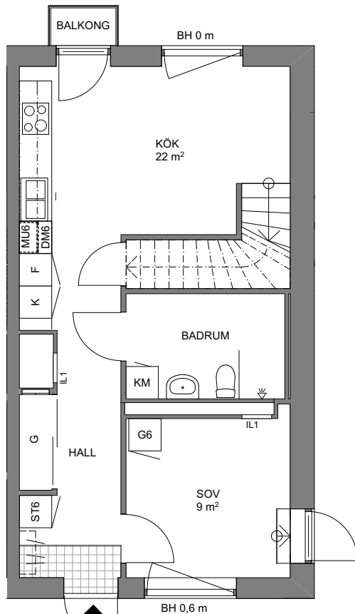
NEDRE PLAN RUMSHÖJD: 2,65 m
