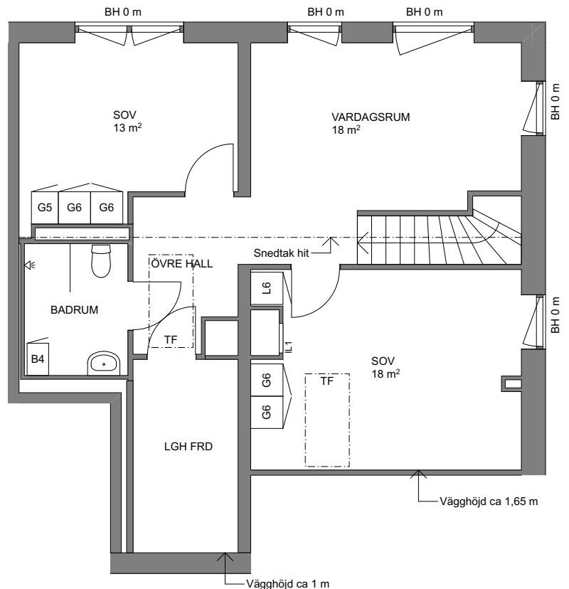
ÖVRE PLAN RUMSHÖJD: CA 3,50m, DELVIS LÄGRE VID SNEDTAK
